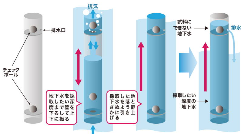
上下のボールが弁となり、筒に取り込んだ水を閉じ込めます
